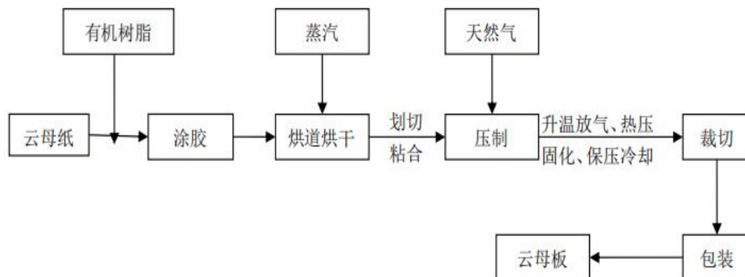
云母板生产工艺流程图
